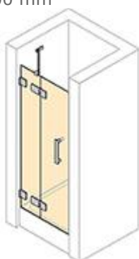
Křídlové dveře s pevným segmentem do niky Šířka: 700 do 1500 mm Výška: 1200 do 2200 mm
