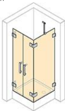
Lítací dveře s boční stěnou Výška: 1200 do 2200 mm Boční stěna: 200 do 1800 mm Dveře: 600 do 1200 mm
