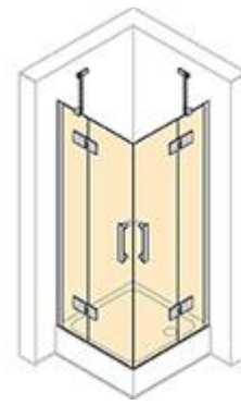
Křídlové dveře s pevnými segmenty jako rohový vstup Šířka: 700 do 1500 mm Výška: 1200 do 2200 mm
