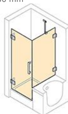
Křídlové dveře s boční stěnou zkrácenou Výška: 1200 do 2200 mm Boční stěna: 200 do 1800 mm Dveře: 500 do 1000 mm
