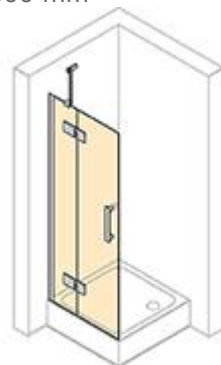
Křídlové dveře s pevným segmentem pro boční stěnu Šířka: 700 do 1500 mm Výška: 1200 do 2200 mm
