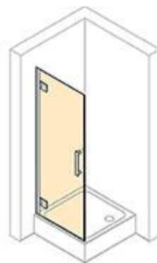
Křídlové dveře pro boční stěnu Šířka: 500 do 1000 mm Výška: 1200 do 2200 mm
