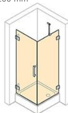
Křídlové dveře s boční stěnou Výška: 1200 do 2200 mm Boční stěna: 200 do 1800 mm Dveře: 500 do 1000 mm
