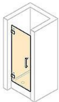
Křídlové dveře do niky Šířka: 500 do 1000 mm Výška: 1200 do 2200 mm
