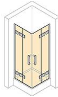
Křídlové sklapovací dveře jako rohový vstup Šířka: 500 do 1250 mm Výška: 1200 do 2000 mm
