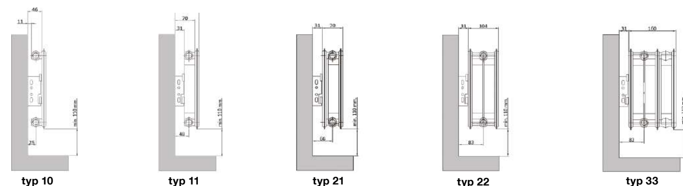
Rozměry panelů radiátoru
