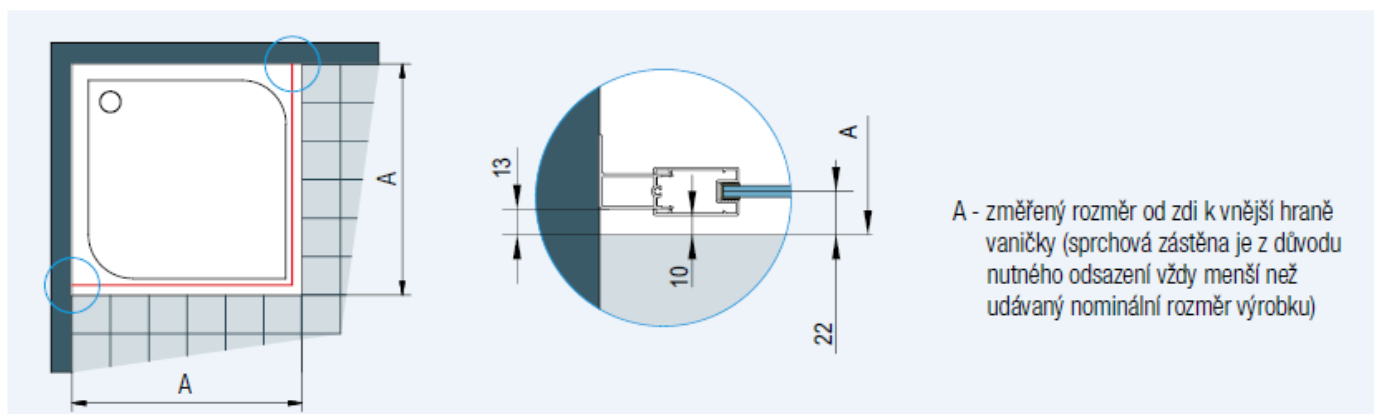
Obr. 1: Při montáži na vaničku je odsazení 13 mm stejné pro standardní i zvláštní rozměry.
